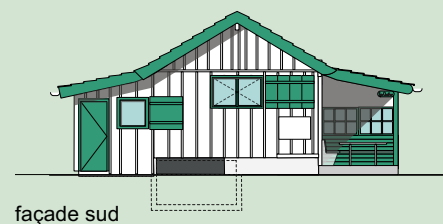
façade sud
