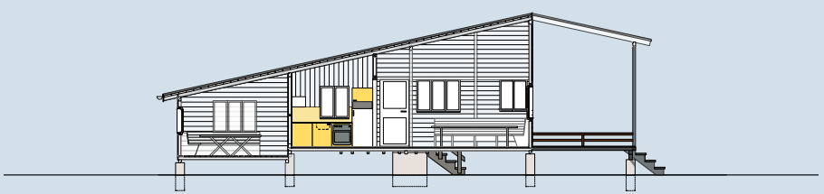
coupe longitudinale
