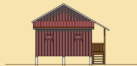
façade sud
