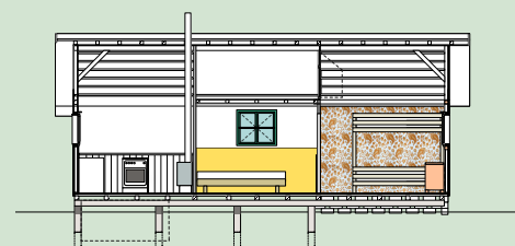
coupe longitudinale
