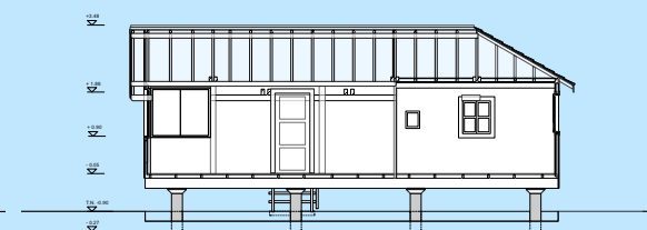
coupe transversale
