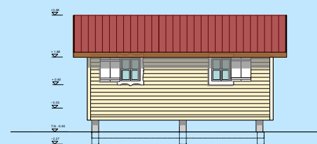
façade sud est
