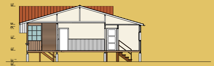
coupe transversale
