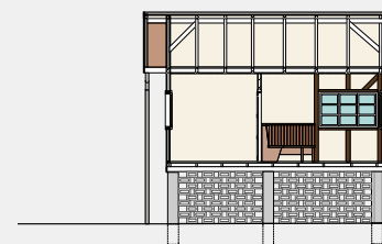
coupe longitudinale
