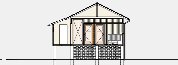
coupe transversale
