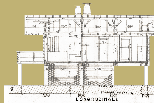
coupe logitudinale
