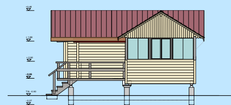
façade nord-ouest
