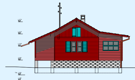
façade sud est
