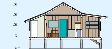
coupe transversale
